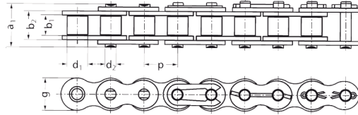
Innen- glied B Außen- glied A Verbindungs- glied mit Feder E Verbindungs- glied mit Splint S
